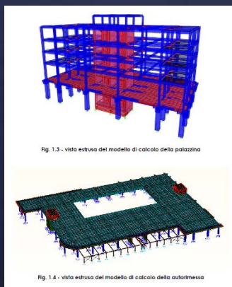
Fig. 1.4 - vista estrusa del modello di calcolo della autorimessa
